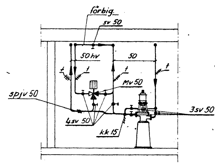
Sektion A-A
